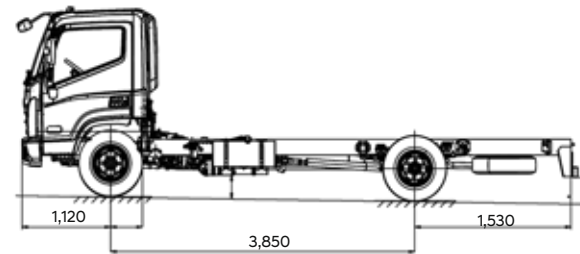
DIMENSIÓN LATERAL
