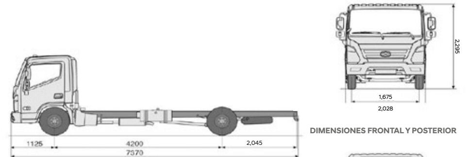
DIMENSIÓN LATERAL
