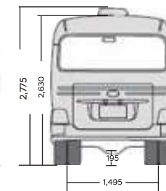
DIMENSIÓN POSTERIOR
